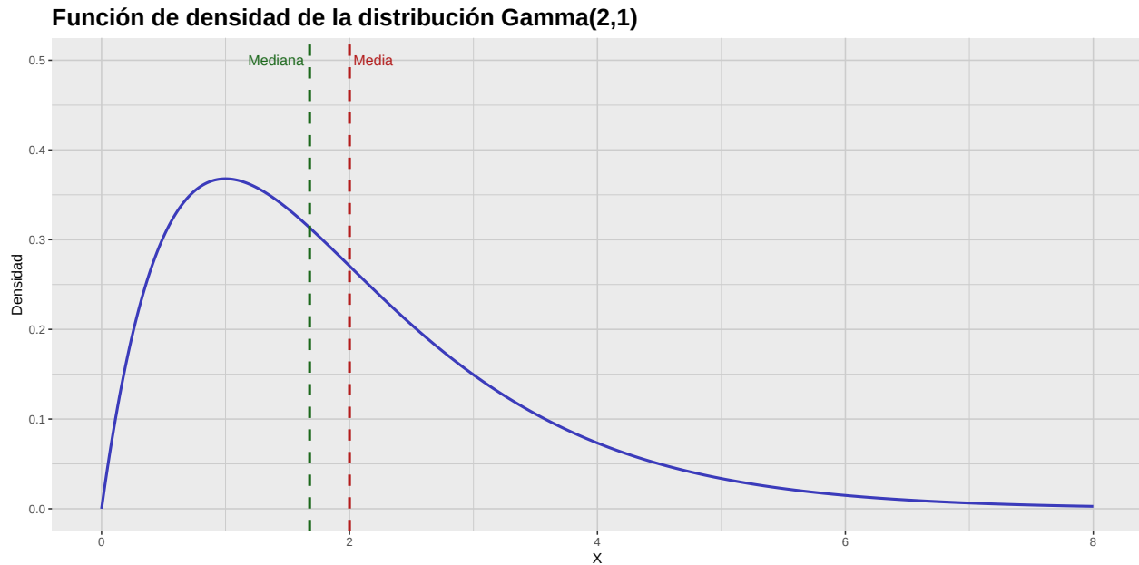
Figura 1.1: Función de densidad de la distribución Gamma con parámetros \alpha = 2 y \beta = 1 . Notemos que para estos parámetros la media es mayor que la mediana, lo cual es común en distribuciones con asimetría positiva.
