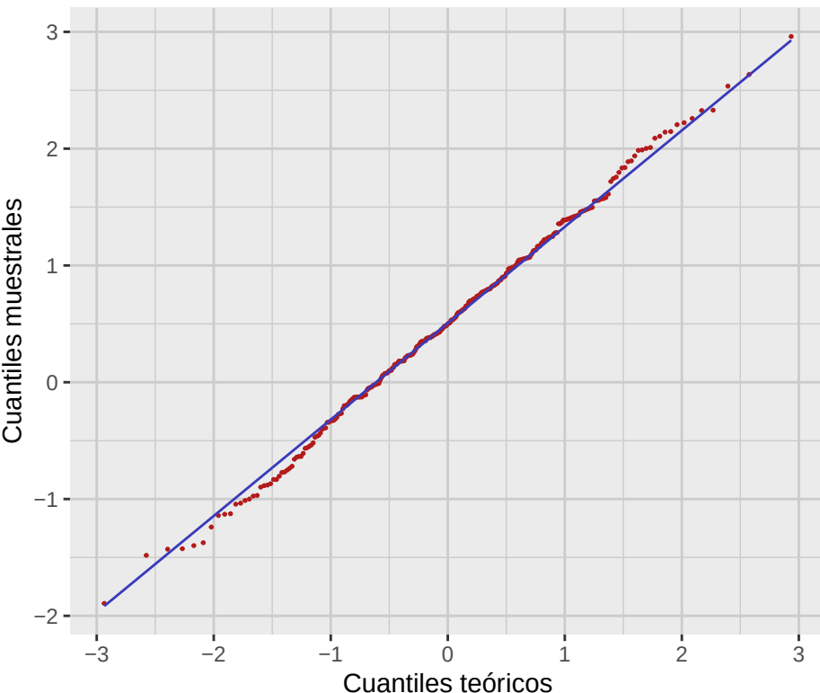
Gráfico QQ
