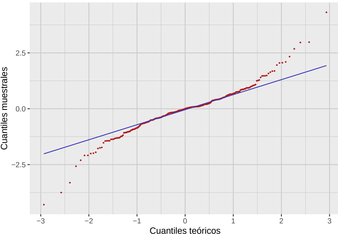
Gráfico QQ
