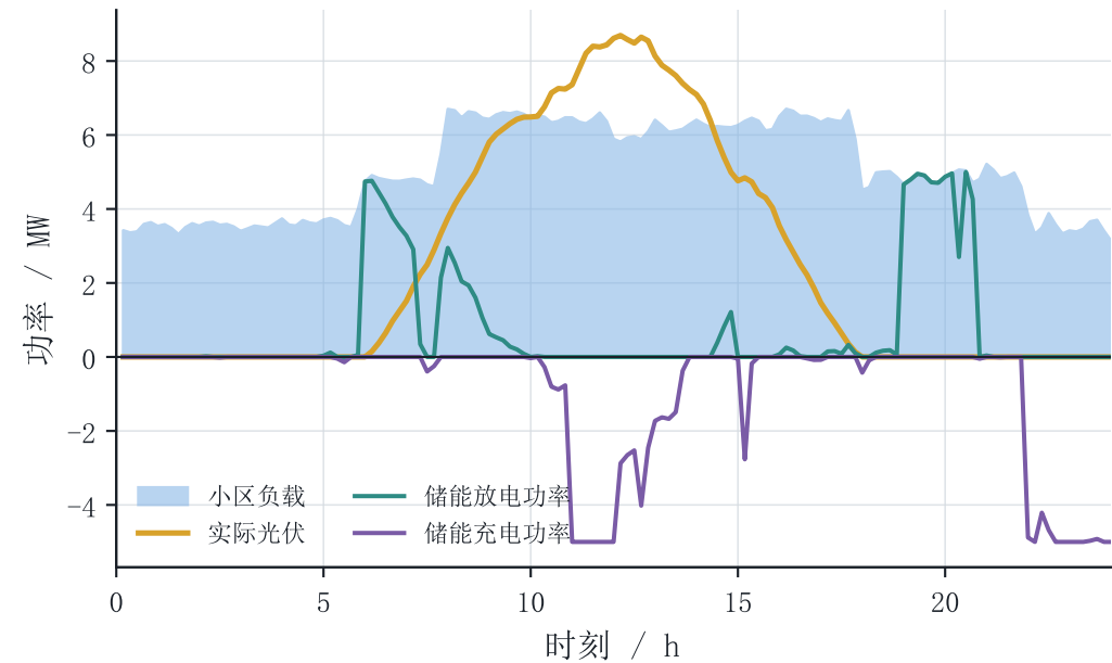
(a) 2025-09-23 功率平衡与储能充放电
