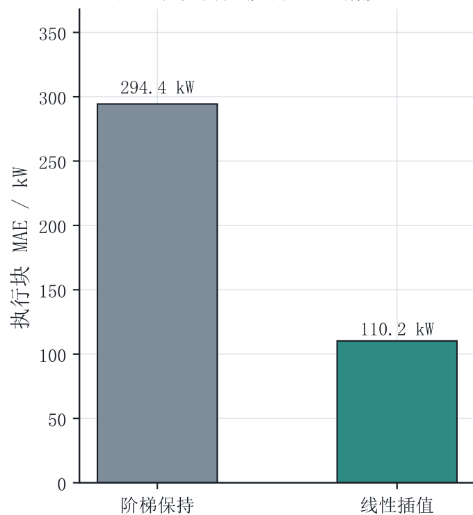
小时预报降尺度方法的精度对比
