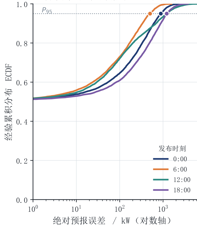
分发布时刻的预报误差累积分布
