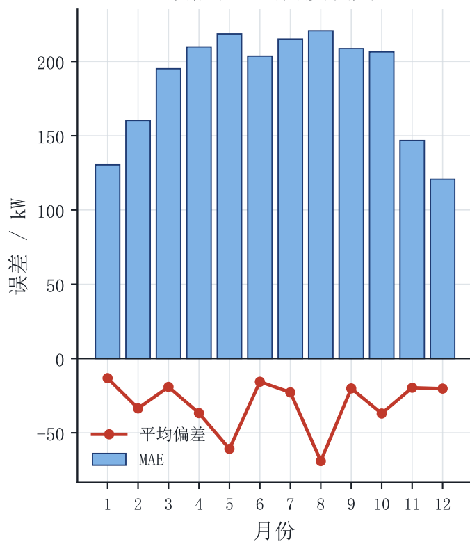
预报误差的月度演变
