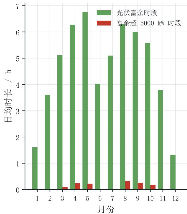
光伏富余的月度强度
