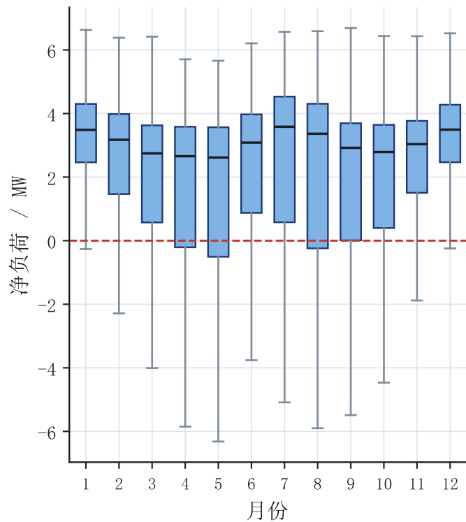
净负荷的月度分布
