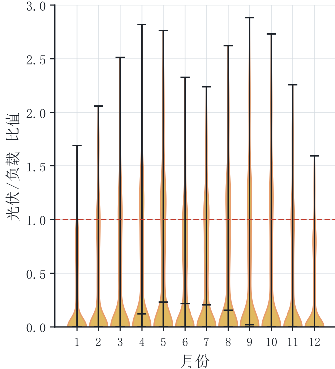
光伏渗透率的月度分布
