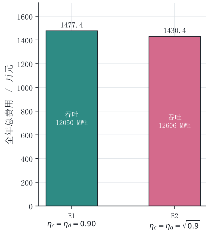
储能效率口径敏感性
