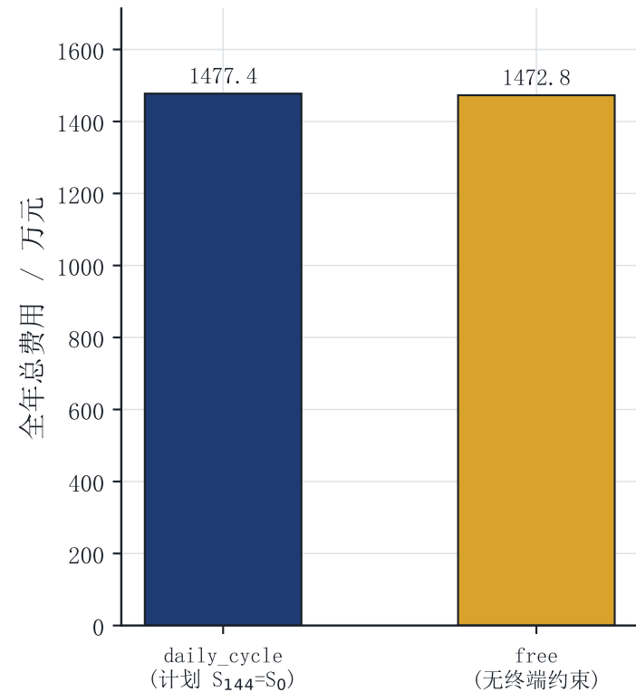
终端储电量策略敏感性
