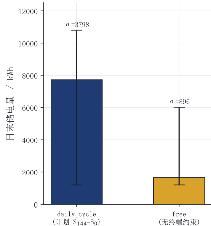
日边界储电量的分布
