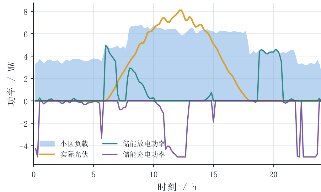
(a) 2025-03-20 功率平衡与储能充放电
