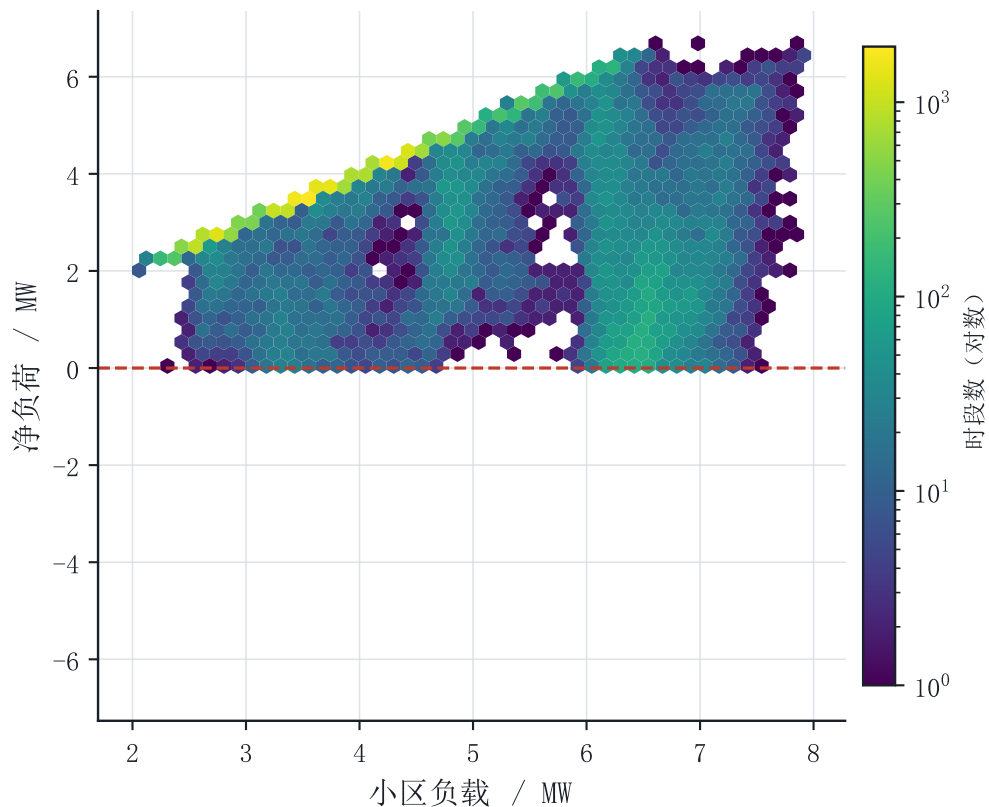
负载—净负荷联合分布（含零线）
