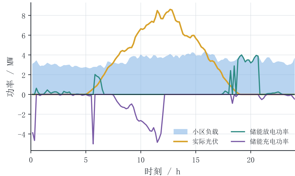
(a) 2025-06-21 功率平衡与储能充放电
