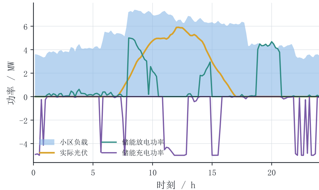
(a) 2025-12-21 功率平衡与储能充放电
