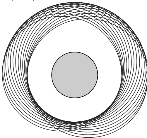
(a) preset drag: orbit trail (rosette)
