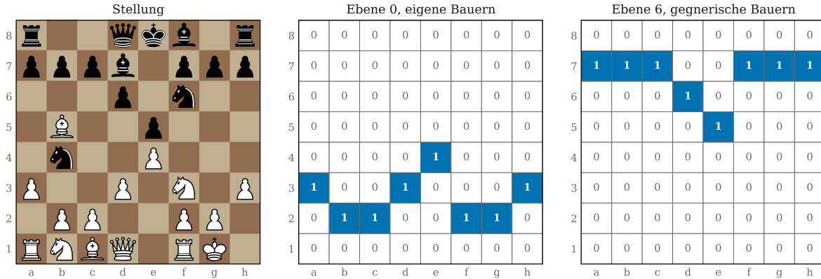
Abbildung 1: Stellung und die zugehörigen Bitboards der Bauern beider Seiten.
