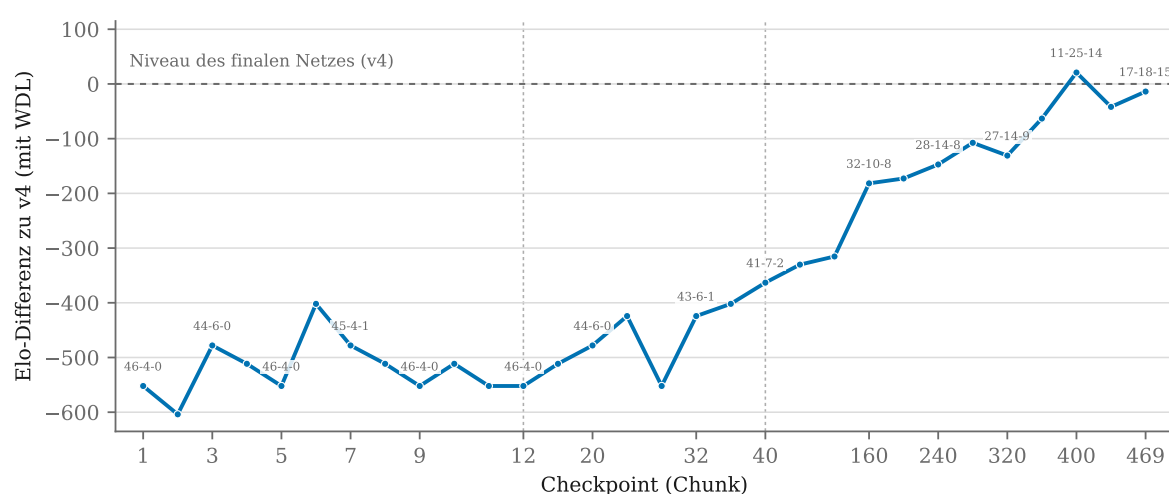
Abbildung 4: Spielstärke der Trainings-Checkpoints von v4 relativ zum fertigen Netz.
