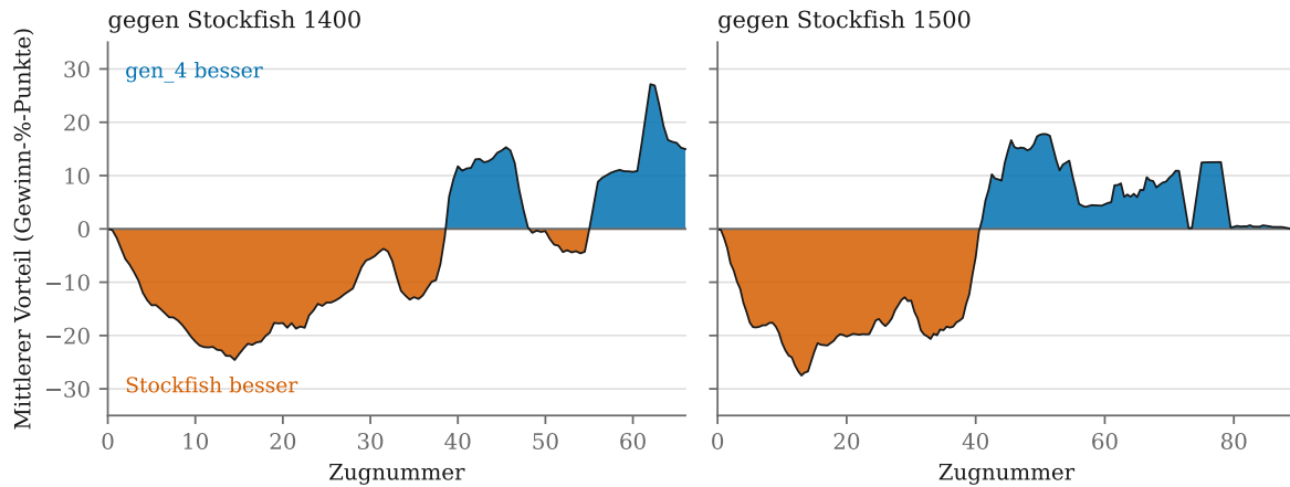
Abbildung 5: Mittlerer Spielverlauf von gen_4 gegen Stockfish 1400 (links) und Stockfish 1500 (rechts) über je zwanzig Partien.
