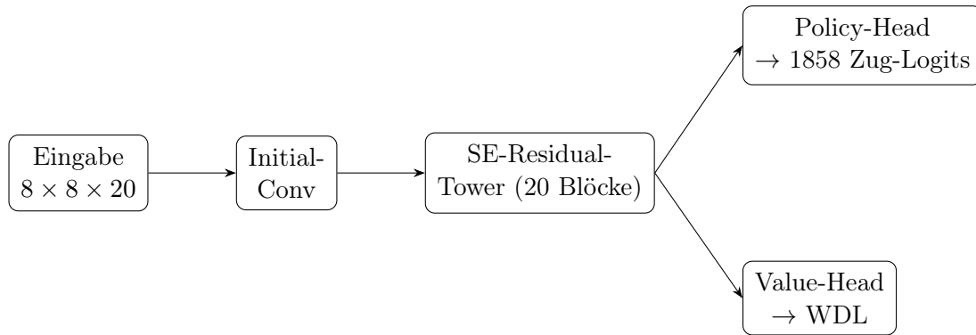
Abbildung 1: Leela-Architektur: geteilter Rumpf, darauf Policy- und Value-Head.
