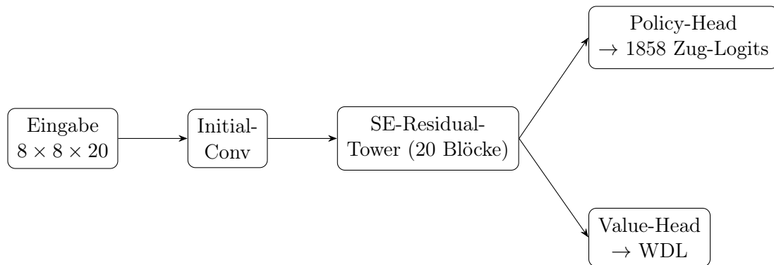
Abbildung 1: Leela-Architektur: geteilter Rumpf, darauf Policy- und Value-Head.
