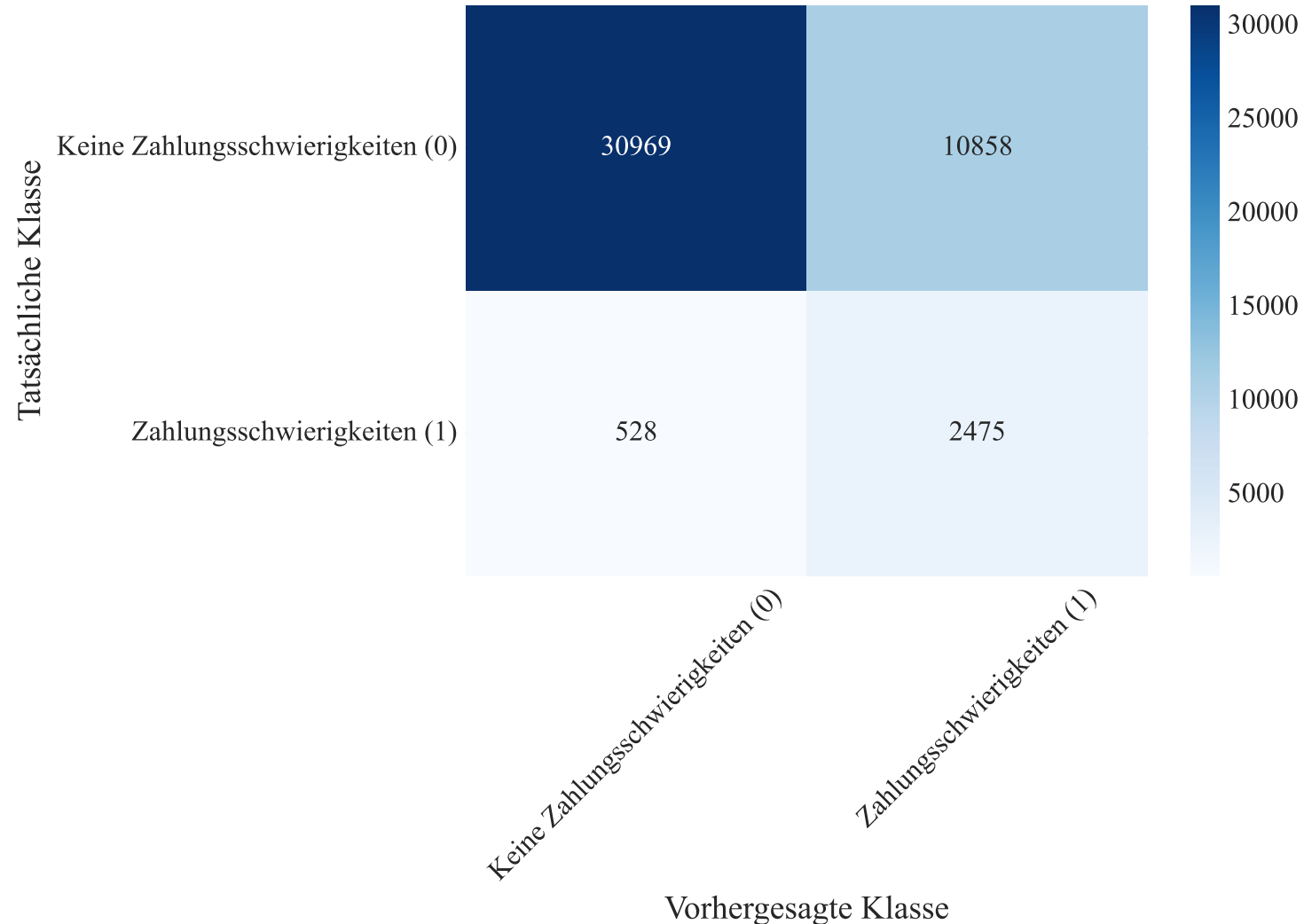
Konfusionsmatrix für LightGBM
