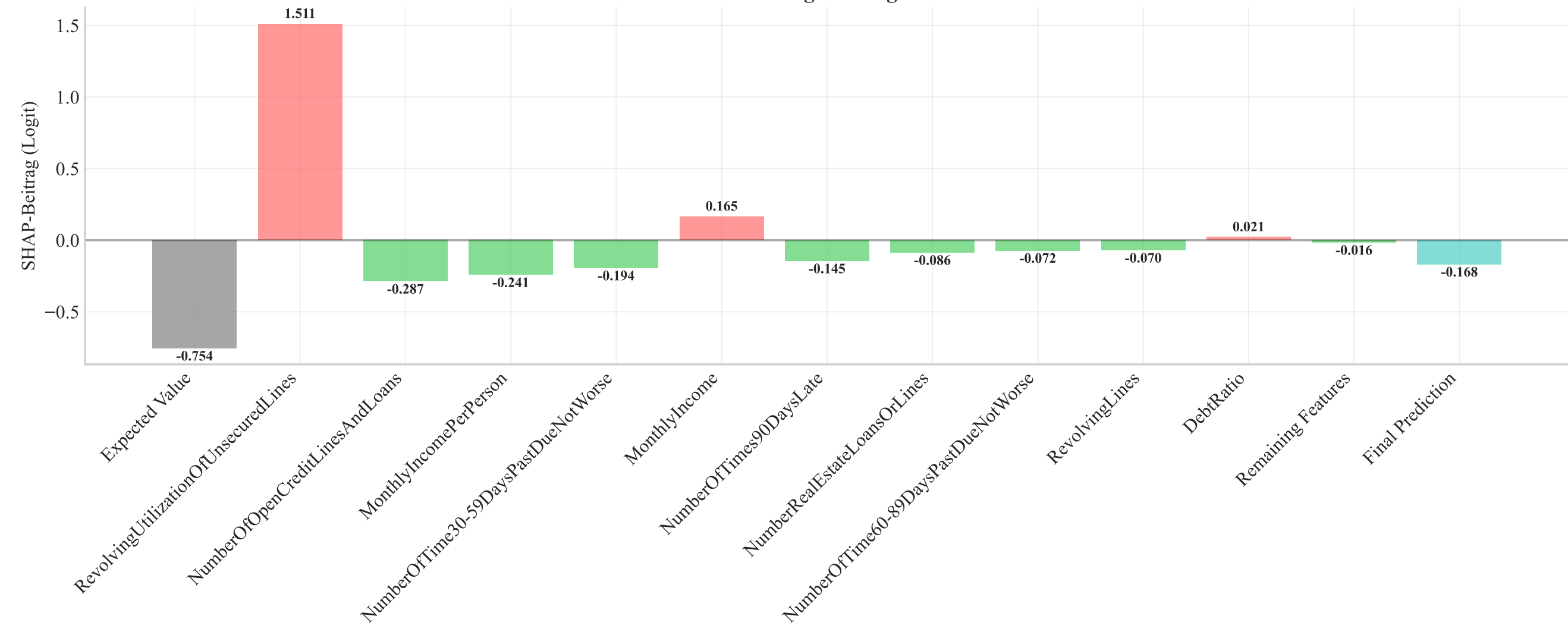
SHAP-Beiträge im Logit-Raum
