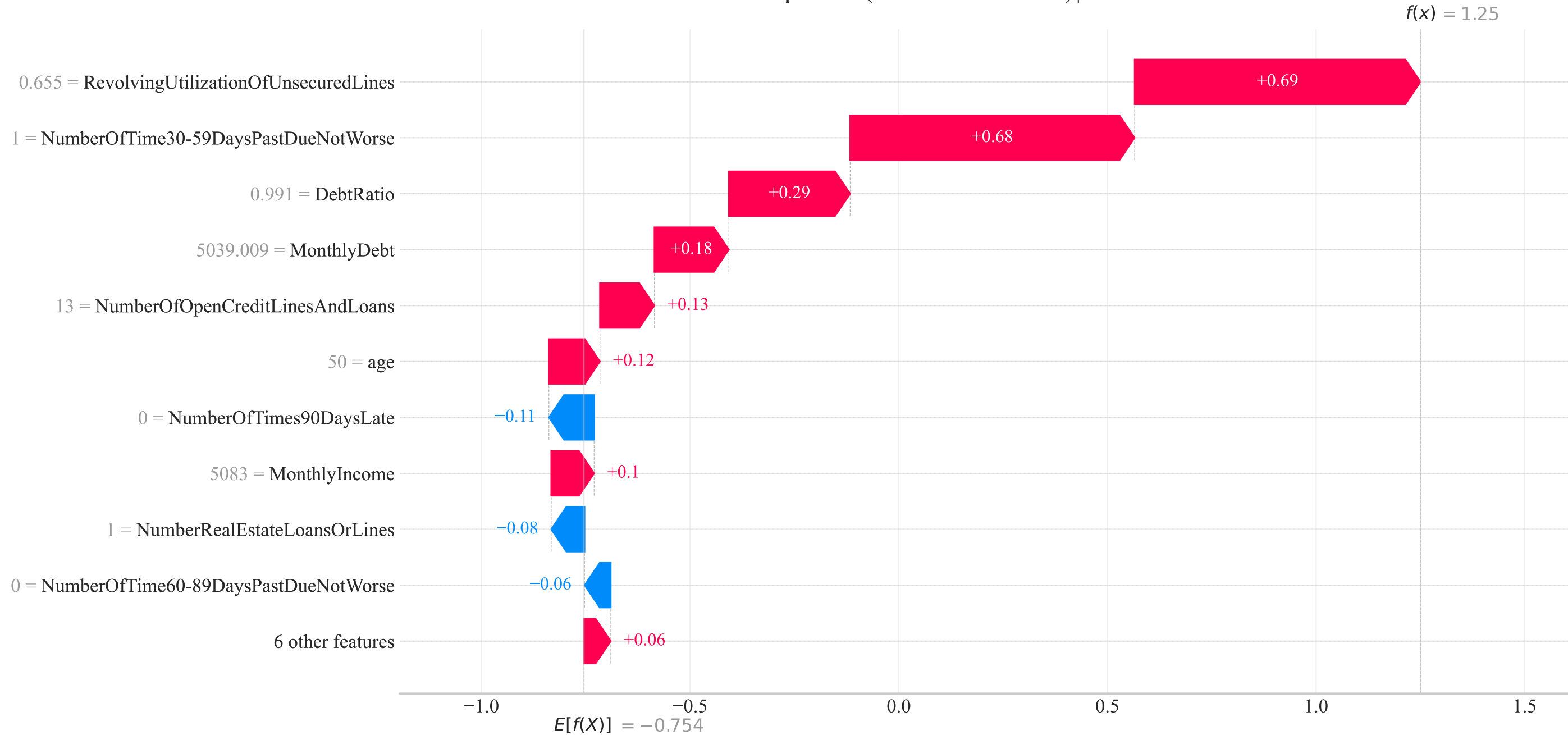
SHAP Waterfall Plot - False Positive Beispiel (Index: 4) Modelloutput: 0.777 (Risikowahrscheinlichkeit) | Tatsächlich: Good Risk
