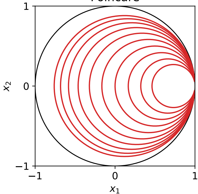
Poincaré
