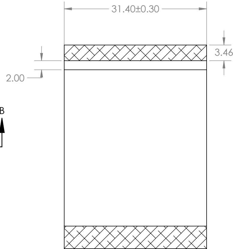
SECTION A-A
