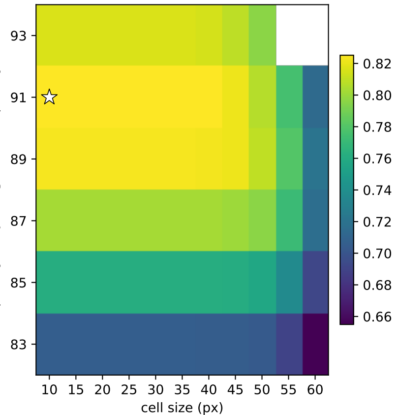
SEG (max = 0.8252 @ 91, 10)
