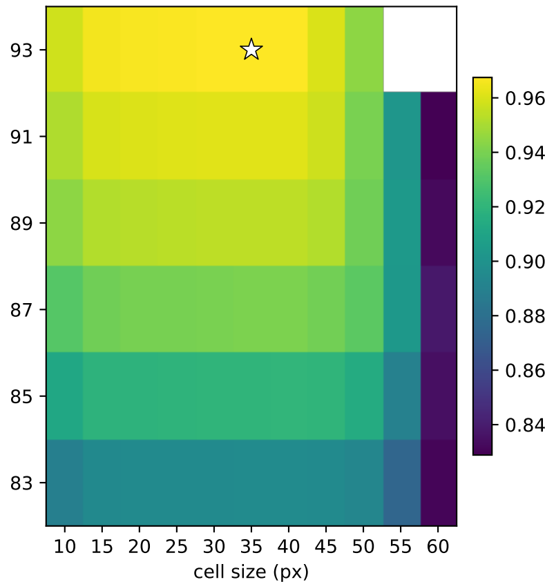
TRA (max = 0.9675 @ 93, 35)
