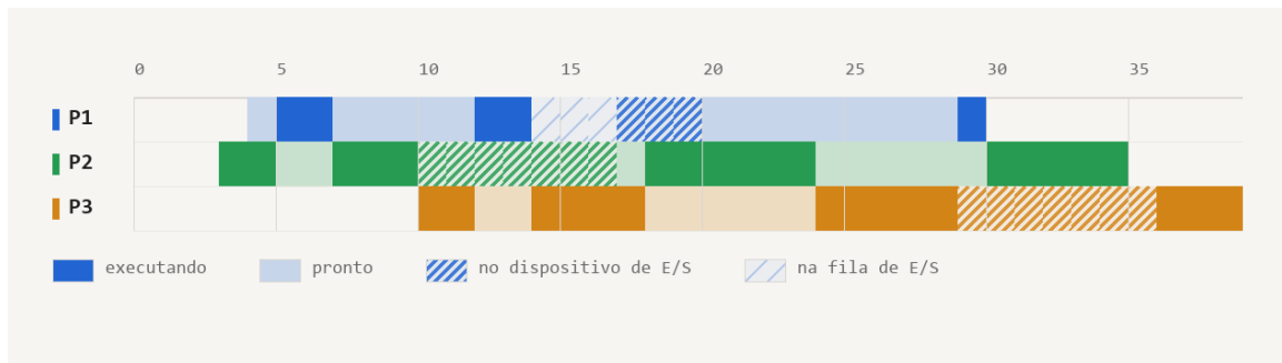
Figura 4: Gráfico de Gantt da execução com o MLFQ.
