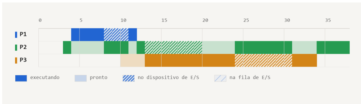
Figura 5: Gráfico de Gantt da execução com o SRTF, sobre os mesmos processos.
