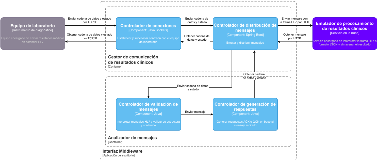
Diagrama de componentes para un sistema de laboratorios clínicos - Interfaz Middleware Diagrama de componentes para el sistema de intercambio de resultados clínicos entre equipos de laboratorio con estándar HL7 y el sistema de comunicación y almacenamiento de mensajes
