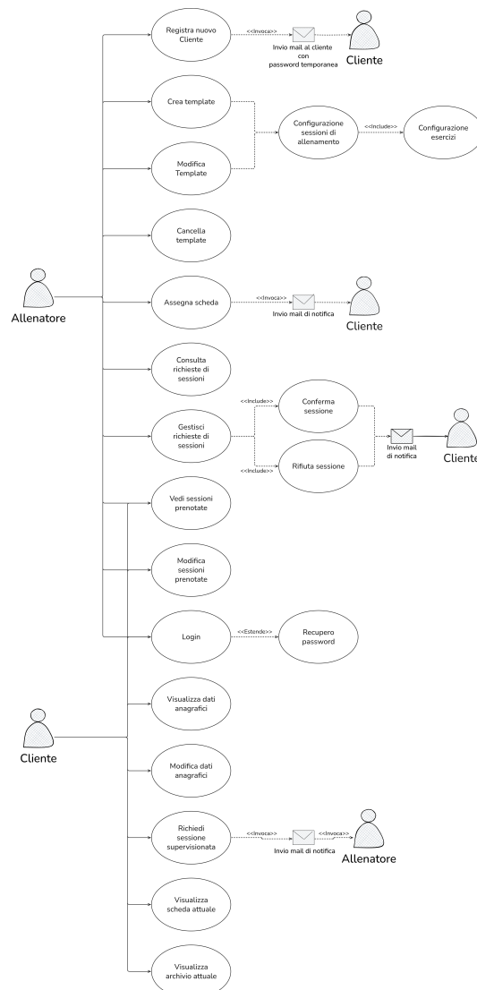
Figura 1: Diagramma dei casi d'uso
