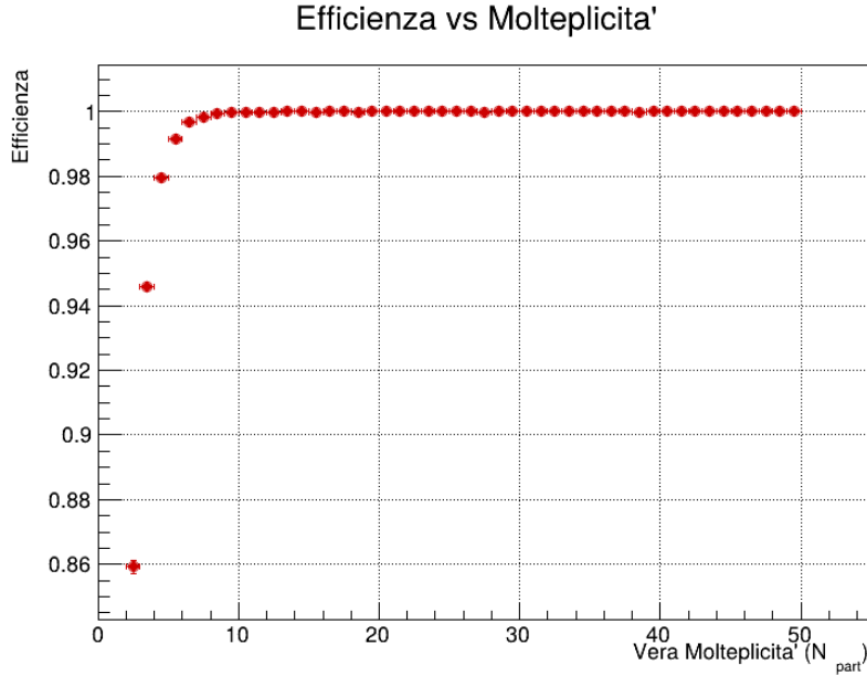
Figura 3: Efficienza di ricostruzione del vertice primario in funzione della molteplicità generata.
