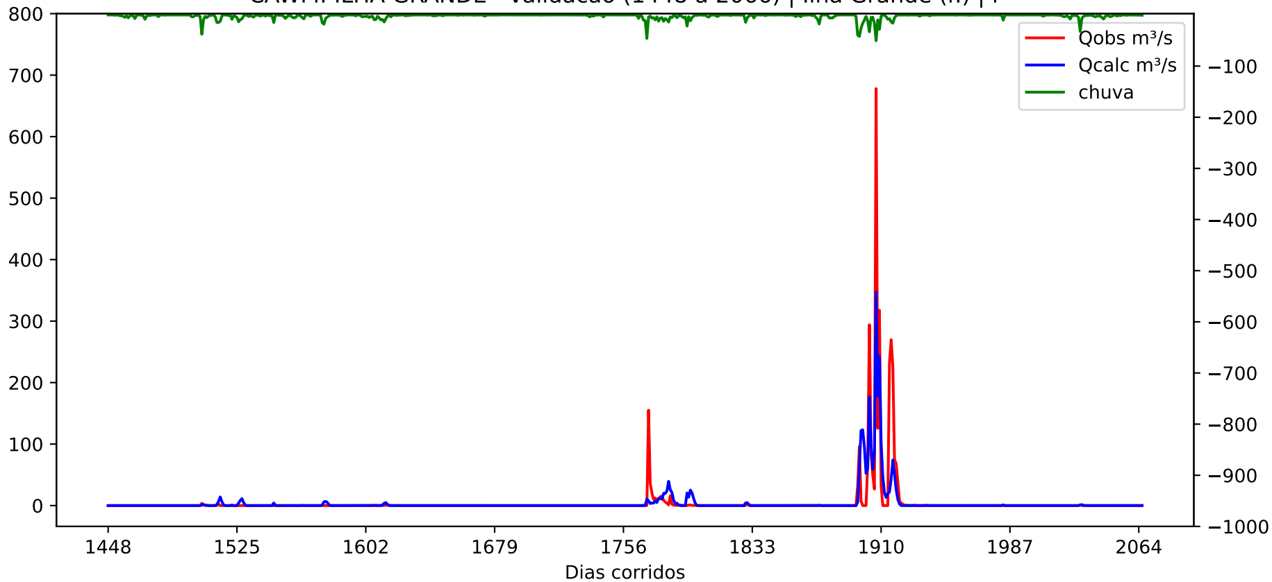
CAWM: ILHA GRANDE - validacao (1448 a 2066) | Ilha Grande (r.) | r
