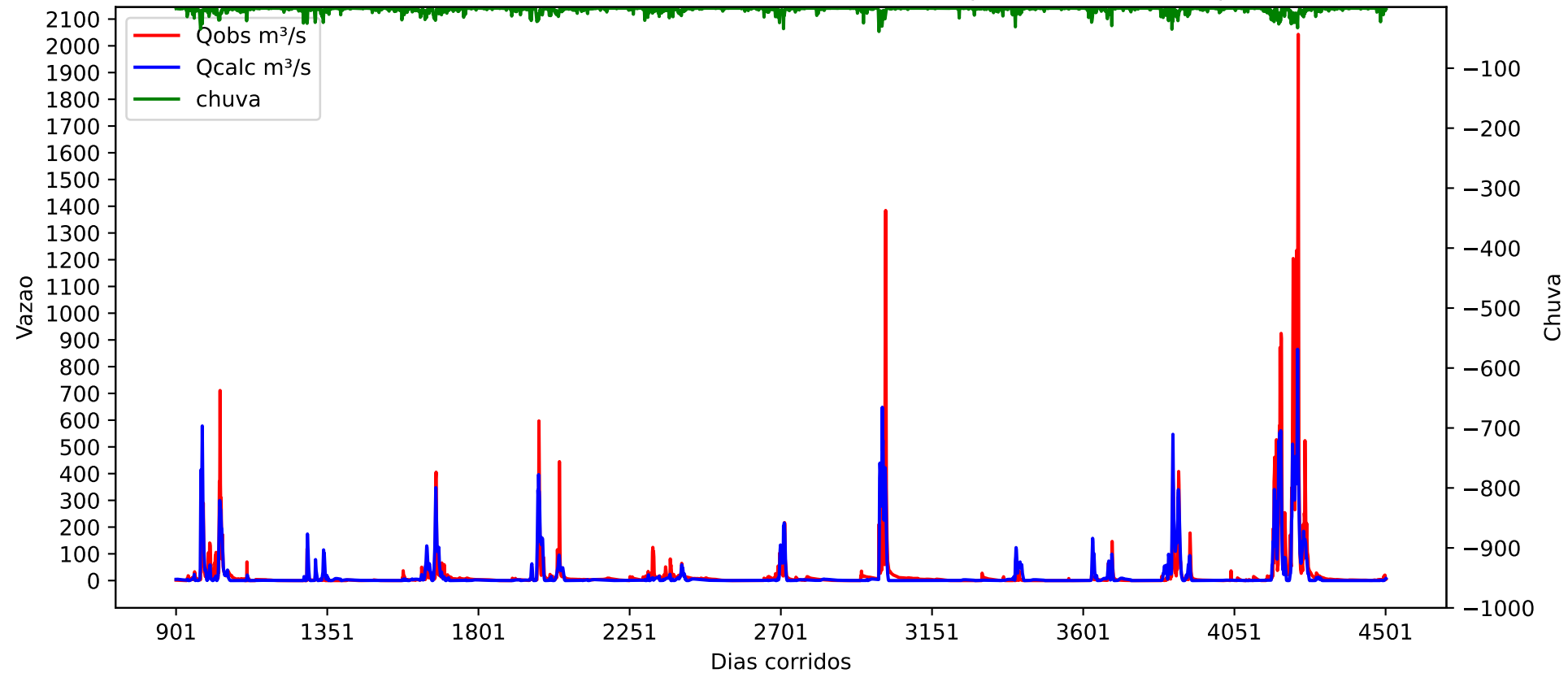
CAWM: SERRA TALHADA - validacao (901 a 4502) | Serra Talhada (r.) | r
