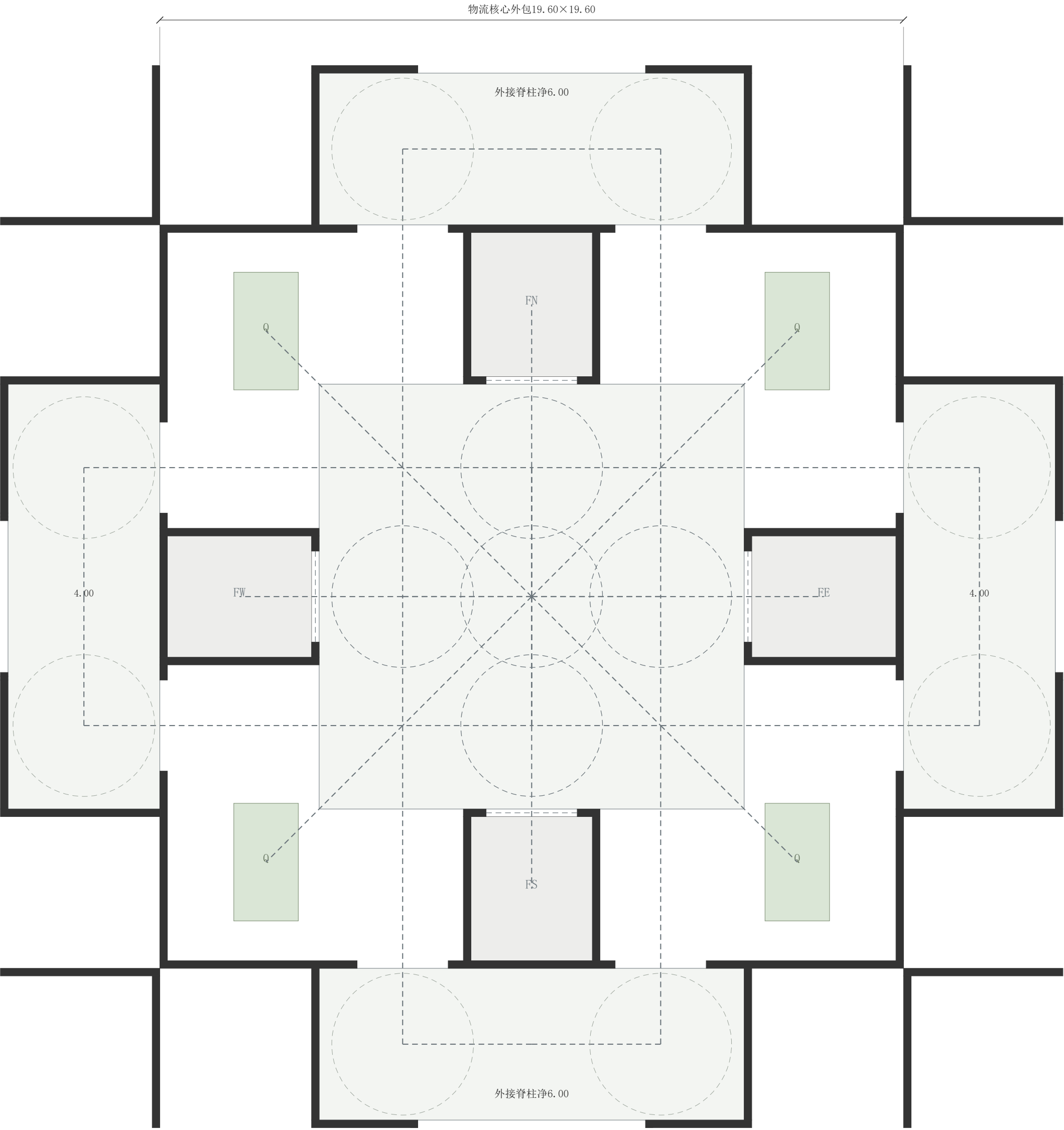
03 中央四货梯 / 原位回转、双侧绕行、四等待位
