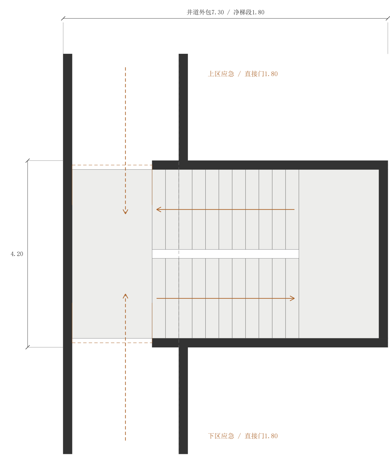
01 左消防楼梯 / 半外置、无额外前室
