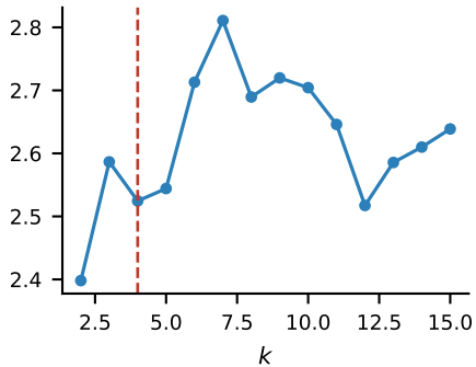
Davies--Bouldin \downarrow
