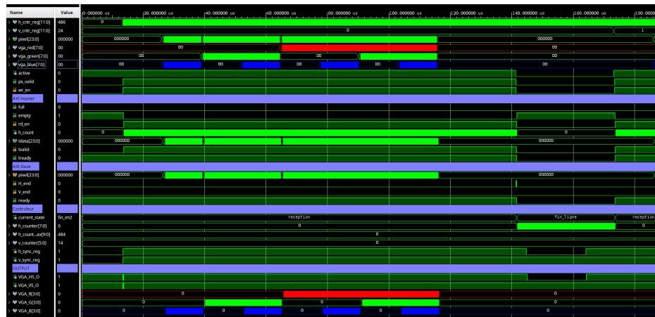
FIG. 6 – TPG vers AXI vers Controleur VGA simulation 1
