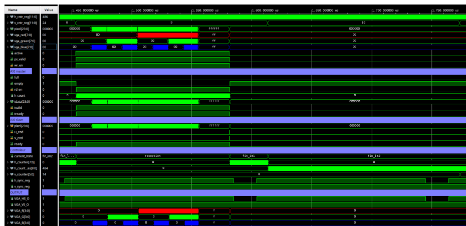
FIG. 8 – TPG vers AXI vers Contrôleur VGA simulation 3
