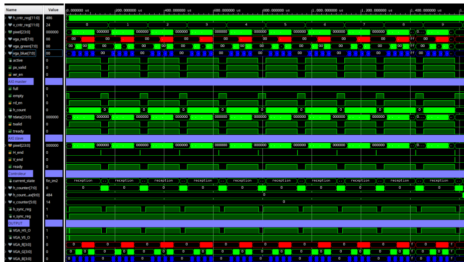
FIG. 7 – TPG vers AXI vers Contrôleur VGA simulation 2
