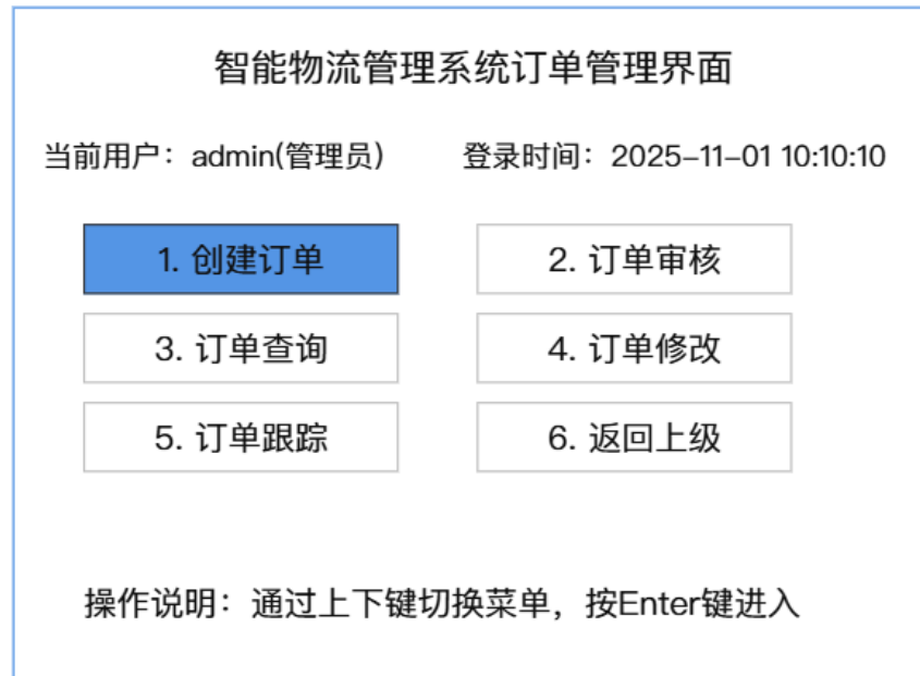
图6 订单管理界面
