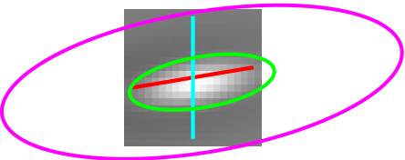
Cell 659 | tau 2.88 Data 90 | Env 10 d 80 FFT 10 d 80
