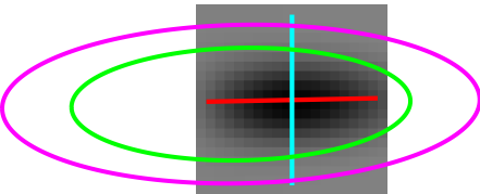
Cell 1430 | tau 3.00 Data 90 | Env 1 d 89 FFT 1 d 89
