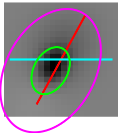
Cell 1852 | tau 1.49 Data 0 | Env 61 d 61 FFT 61 d 61
