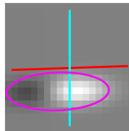
Cell 1645 | tau 2.70 Data 90 | Env 2 d 88 FFT 2 d 88
