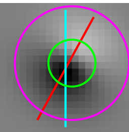
Cell 121 | tau 1.00 Data 90 | Env 61 d 29 FFT 61 d 29
