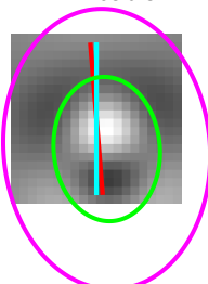
Cell 244 | tau 1.36 Data 90 | Env 95 d 5 FFT 95 d 5
