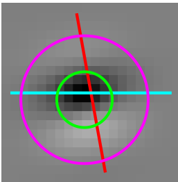
Cell 1589 | tau 1.00 Data 0 | Env 100 d 80 FFT 100 d 80
