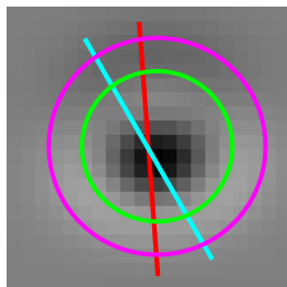
Cell 1644 | tau 1.00 Data 120 | Env 94 d 26 FFT 94 d 26
