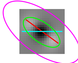
Cell 798 | tau 2.17 Data 0 | Env 144 d 36 FFT 144 d 36
