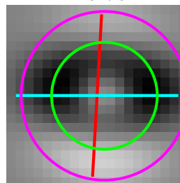
Cell 1762 | tau 1.01 Data 0 | Env 87 d 87 FFT 87 d 87
