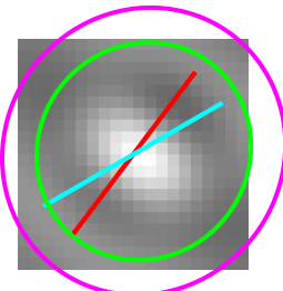
Cell 614 | tau 1.05 Data 30 | Env 53 d 23 FFT 53 d 23
