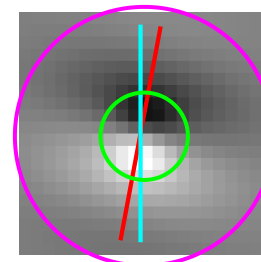
Cell 629 | tau 1.00 Data 90 | Env 79 d 11 FFT 79 d 11
