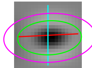
Cell 123 | tau 1.86 Data 90 | Env 3 d 87 FFT 3 d 87
