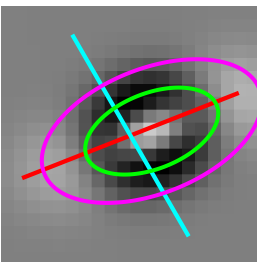
Cell 1608 | tau 1.85 Data 120 | Env 21 d 81 FFT 21 d 81
