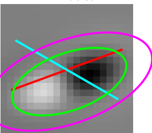
Cell 1832 | tau 2.09 Data 150 | Env 20 d 50 FFT 20 d 50
