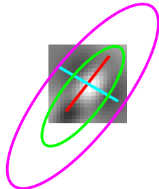
Cell 775 | tau 3.00 Data 150 | Env 52 d 82 FFT 52 d 82
