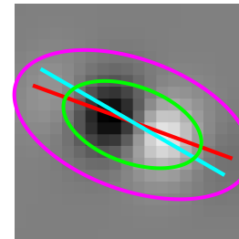
Cell 1601 | tau 1.89 Data 150 | Env 160 d 10 FFT 160 d 10
