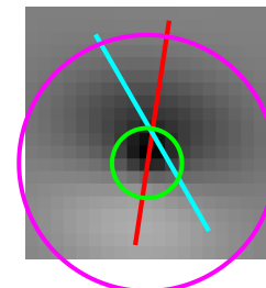
Cell 1614 | tau 1.00 Data 120 | Env 81 d 39 FFT 81 d 39
