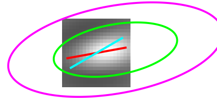
Cell 1431 | tau 2.49 Data 30 | Env 10 d 20 FFT 10 d 20
