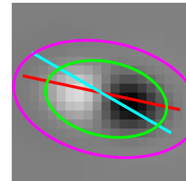
Cell 1641 | tau 1.66 Data 150 | Env 168 d 18 FFT 168 d 18
