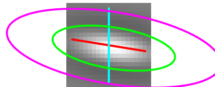
Cell 1833 | tau 3.00 Data 90 | Env 171 d 81 FFT 171 d 81
