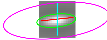
Cell 870 | tau 3.00 Data 90 | Env 6 d 84 FFT 6 d 84
