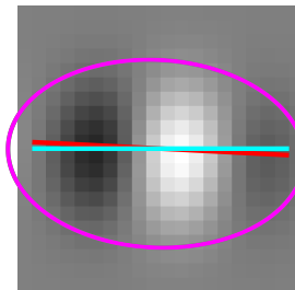
Cell 1861 | tau 1.58 Data 0 | Env 177 d 3 FFT 177 d 3
