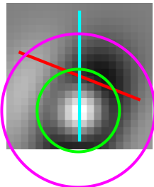
Cell 1453 | tau 1.00 Data 90 | Env 158 d 68 FFT 158 d 68
