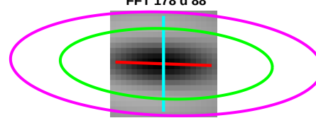
Cell 744 | tau 3.00 Data 90 | Env 178 d 88 FFT 178 d 88
