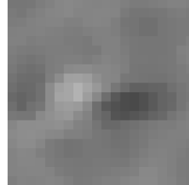
Cell 1641 DSI 0.25 | OSI 0.92
