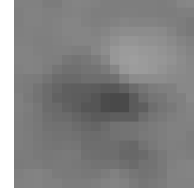
Cell 121 DSI 0.29 | OSI 0.58
