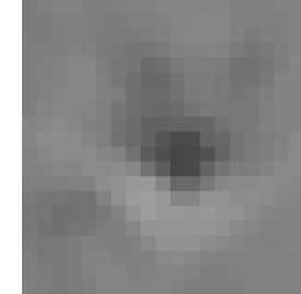
Cell 130 DSI 0.74 | OSI 1.00
