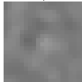
Cell 362 DSI 0.24 | OSI 0.19
