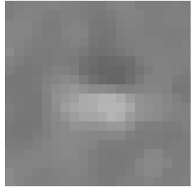
Cell 250 DSI 0.77 | OSI 1.00
