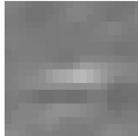
Cell 1847 DSI 0.73 | OSI 1.00
