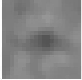
Cell 123 DSI 0.26 | OSI 1.00
