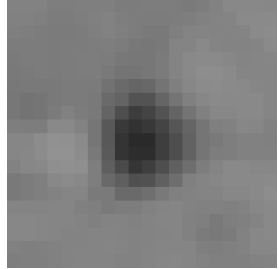
Cell 131 DSI 0.47 | OSI 0.96
