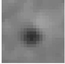
Cell 94 DSI 0.04 | OSI 0.18
