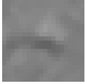
Cell 140 DSI 1.00 | OSI 1.00
