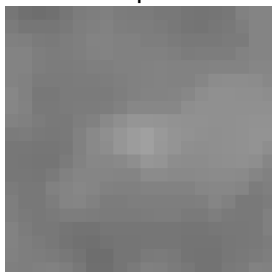
Cell 1431 DSI 0.18 | OSI 0.51
