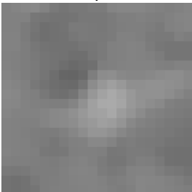
Cell 1546 DSI 1.00 | OSI 0.05
