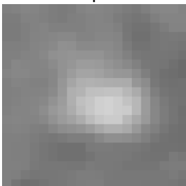
Cell 1422 DSI 0.06 | OSI 0.57
