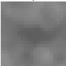
Cell 1430 DSI 0.05 | OSI 0.73
