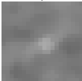
Cell 775 DSI 0.23 | OSI 0.84
