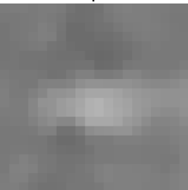
Cell 95 DSI 0.31 | OSI 1.00
