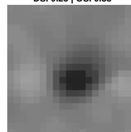
Cell 1815 DSI 0.25 | OSI 0.35
