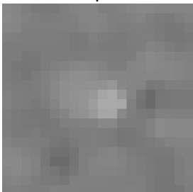
Cell 127 DSI 0.27 | OSI 0.99
