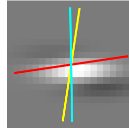
Cell 1847 Data 91 | Env 8 d 83 FFT 82 d 9
