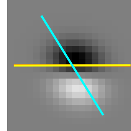
Cell 808 Data 122 | Env 180 d 58 FFT 0 d 58
