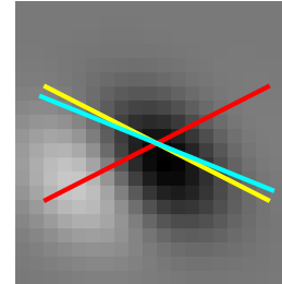
Cell 1642 Data 158 | Env 27 d 49 FFT 153 d 5
