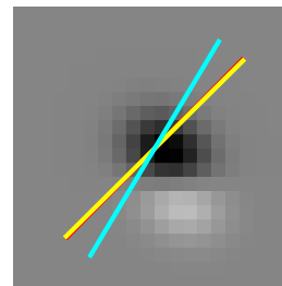
Cell 1086 Data 59 | Env 45 d 14 FFT 45 d 14
