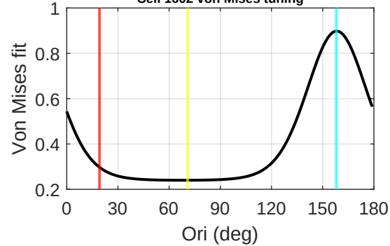
Cell 1602 von Mises tuning
