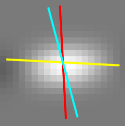
Cell 1517 Data 105 | Env 93 d 12 FFT 177 d 72
