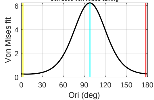
Cell 1606 von Mises tuning
