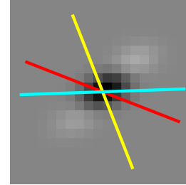
Cell 1510 Data 2 | Env 159 d 23 FFT 111 d 71
