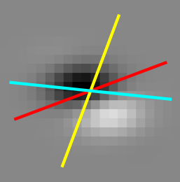
Cell 1828 Data 174 | Env 21 d 27 FFT 69 d 75
