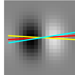
Cell 1622 Data 9 | Env 3 d 6 FFT 177 d 12
