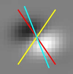
Cell 1563 Data 112 | Env 125 d 13 FFT 55 d 57
