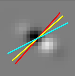
Cell 1620 Data 27 | Env 49 d 22 FFT 41 d 14
