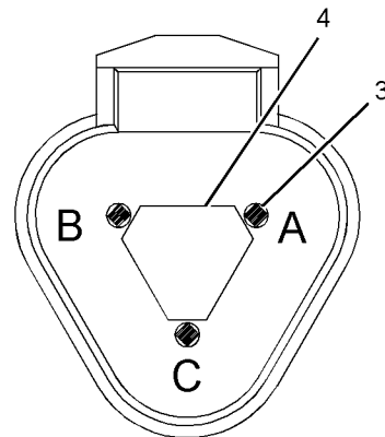
VIEW A-A
