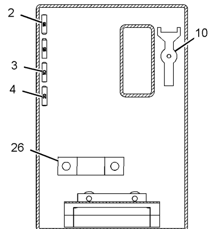
SECTION D-D
