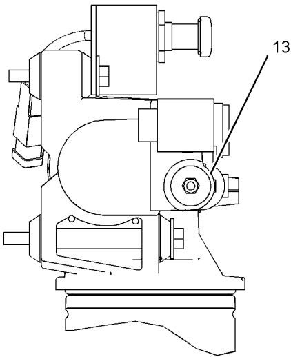
VIEW A-A
