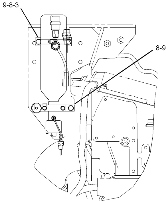
VIEW A-A
