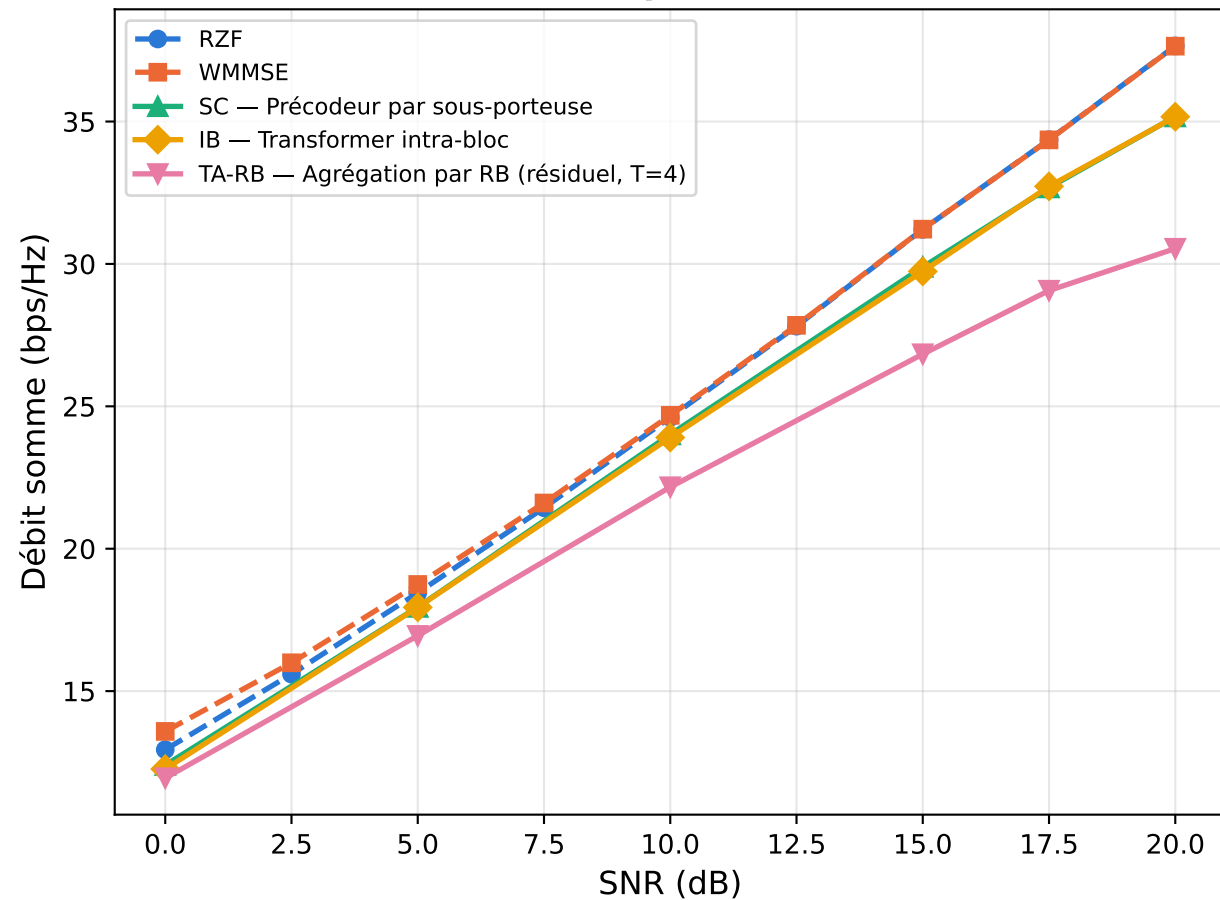
CSI parfait
