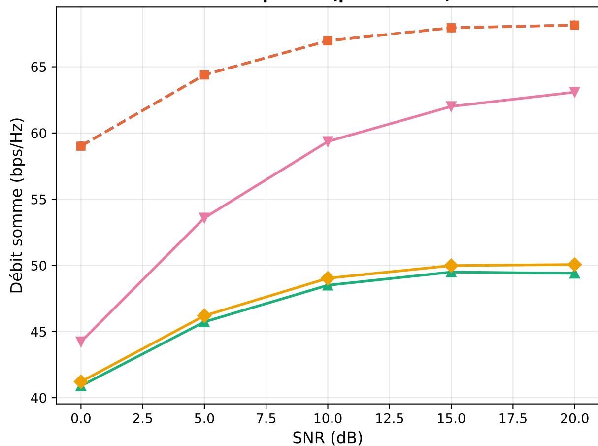
CSI imparfait (pilote 20dB)
