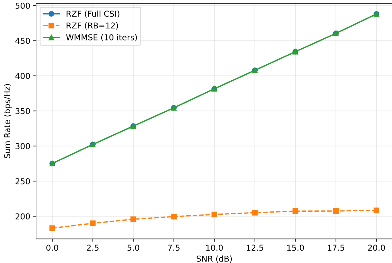
M64K32: RZF vs WMMSE
