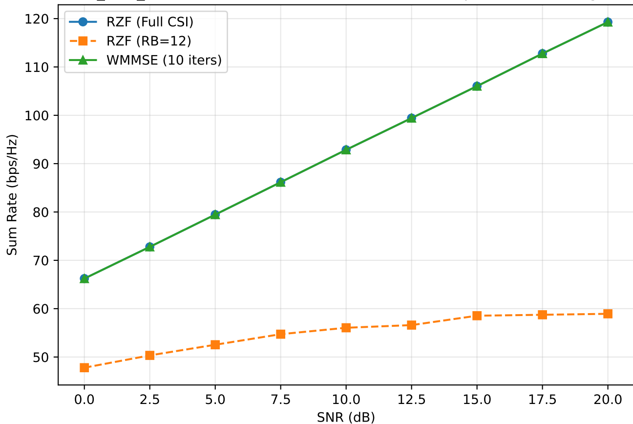
M64K8_true_uma: RZF vs WMMSE (canal STANDARD, pas de clustering forcé)
