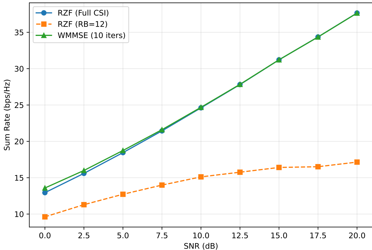
M8K4 (UMa): RZF vs WMMSE
