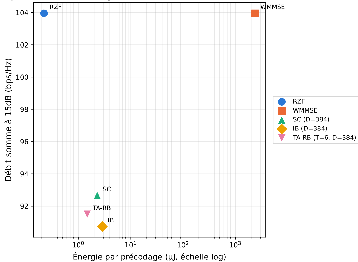
Compromis débit / énergie — UMi MASSIVE (M=64, K=8), D=384
