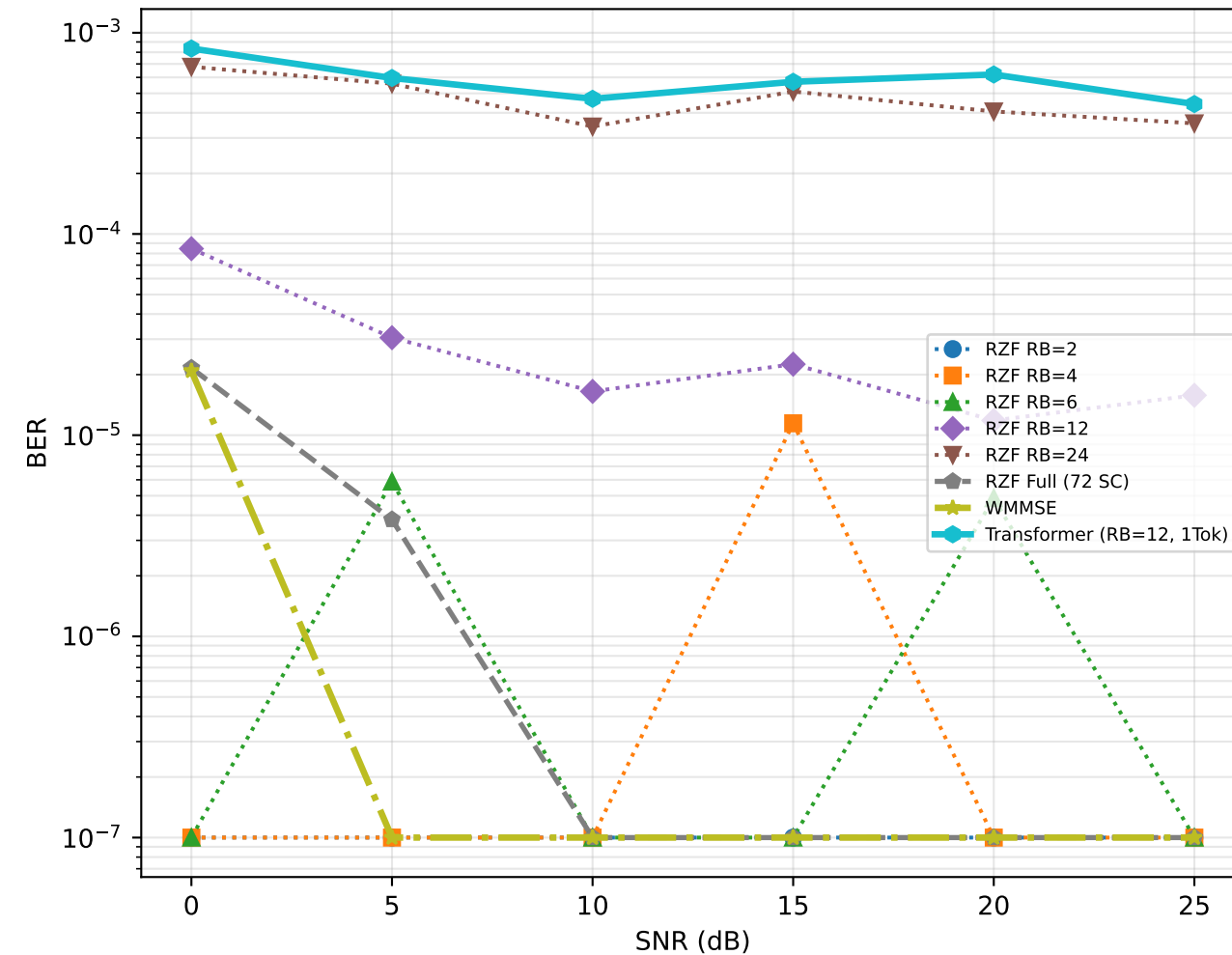
(b) BER
