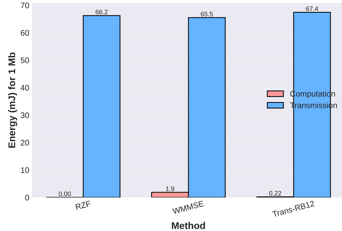
(d) Energy Breakdown @ 15 dB SNR
