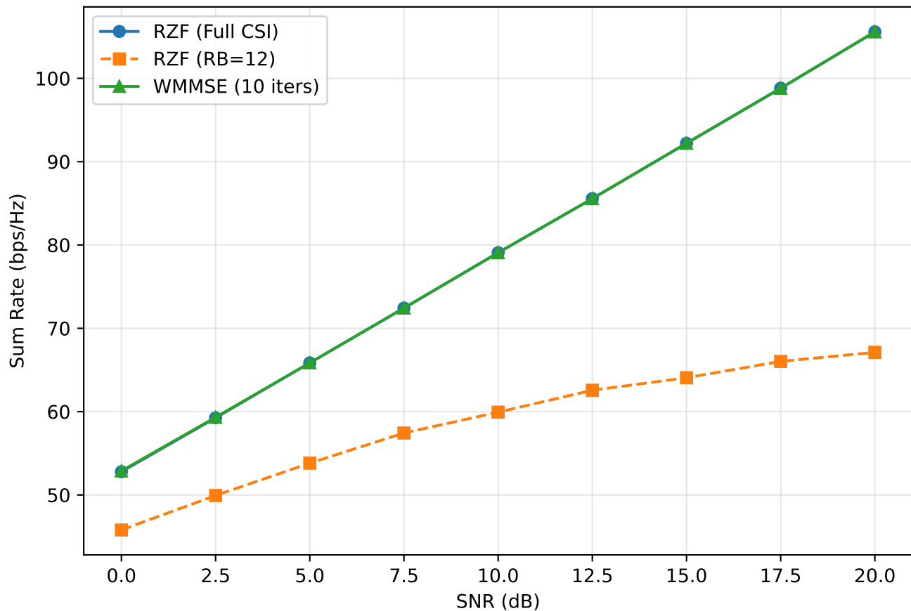
M32K8: RZF vs WMMSE
