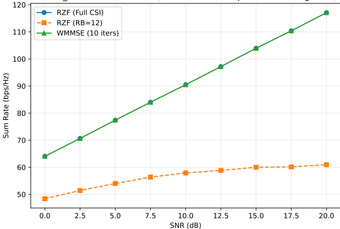
M64K8_true: RZF vs WMMSE (canal STANDARD, pas de clustering forcé)
